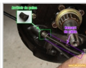
Arrêteur de gaine et ressort de câbles
